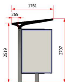
Marquesina Solarium Medidas generales (1:50)
